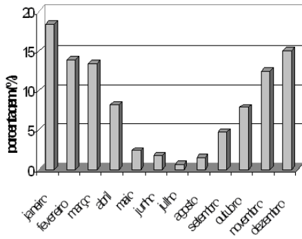
Figura 2: Histograma de porcentagem da altura pluviométrica acumulada mensal em Santo Antônio de Lerveger (1987 a 2006)
