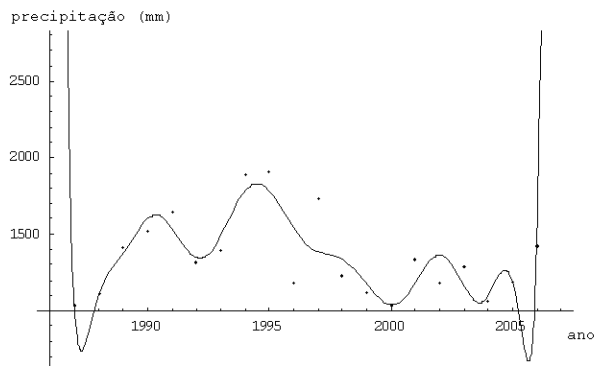
Figura 5: Curva de ajuste pela série de Fourier para a precipitação acumulada de Santo Antônio de Lerveger (1987-2006) – fonte: Prof. Dr. José Holanda Campelo Jr.
