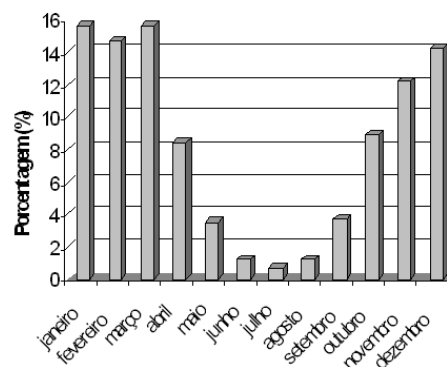
Figura 1: Histograma de porcentagem da altura pluviométrica acumulada mensal em Cuiabá (1912 a 2006)
