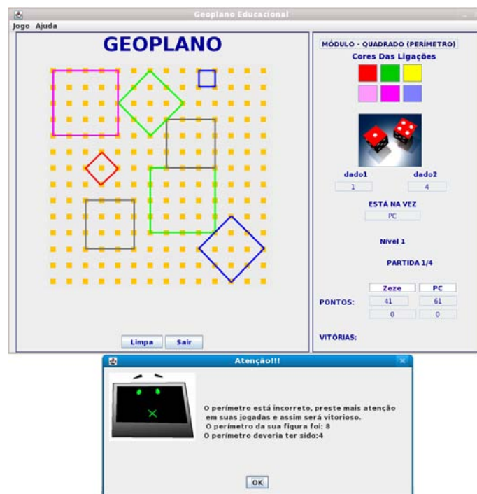
Figura 1: Jogo GeoplanoPEC em execução.
